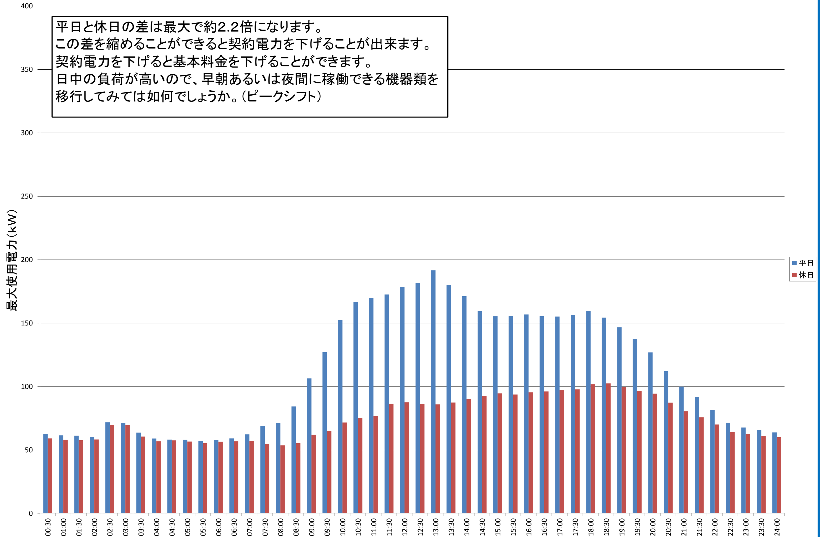
本荘南キャンパス 1月の時間帯別最大使用電力平均値
