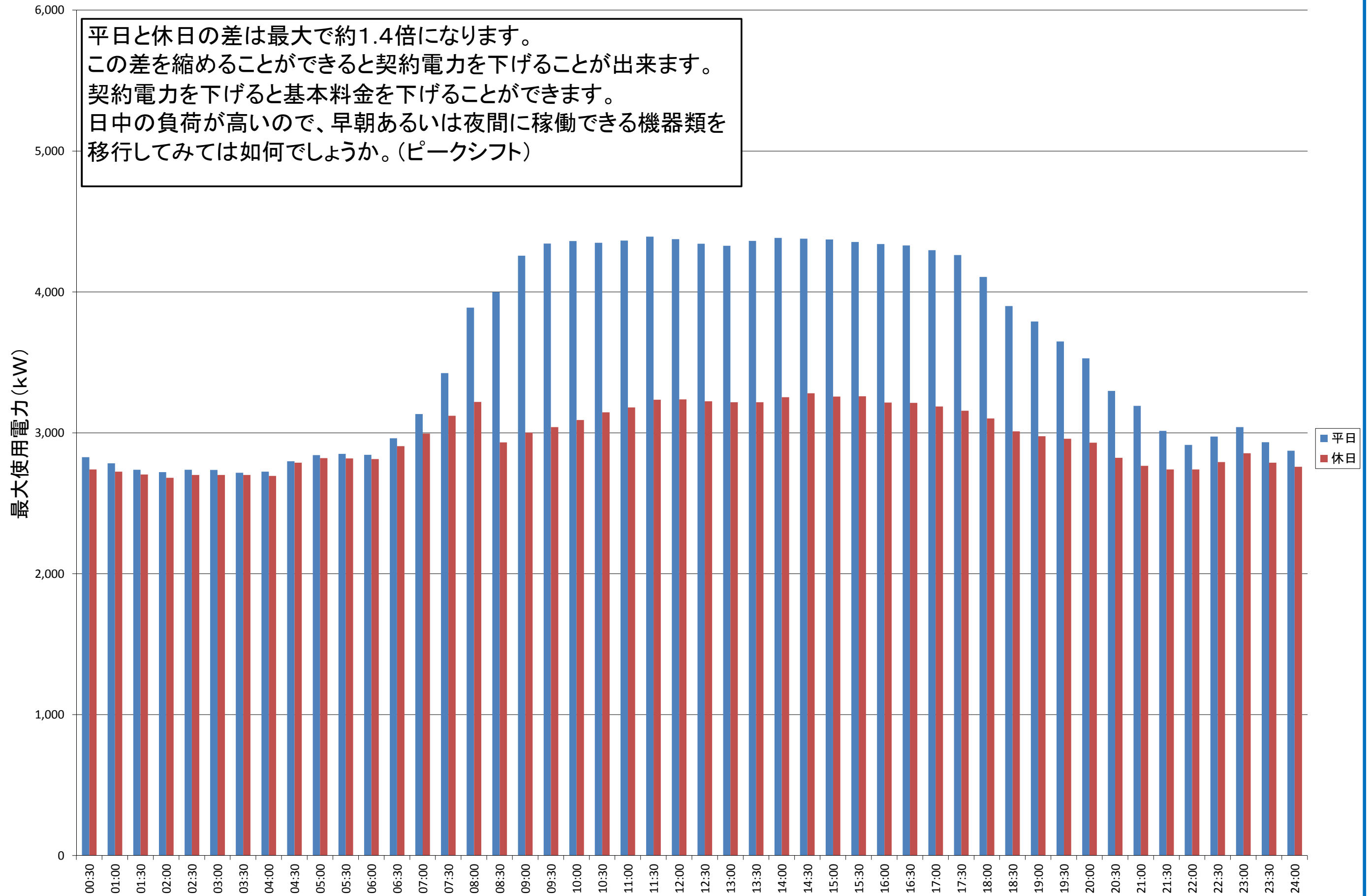
本荘北キャンパス 9月の時間帯別最大使用電力平均値
