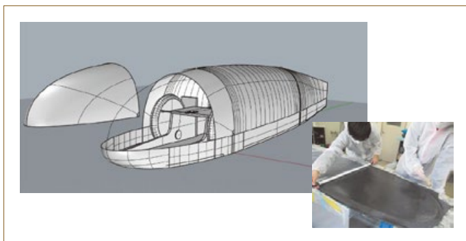
新車両の構想です。電池の消費を抑えるため、空気抵抗の少ない流線形の車両を設計しています。来年のレースまでの完成を目指します。
